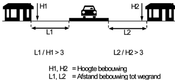
Figuur 18: Schematisch overzicht toepassingsbereik SRM-2.
